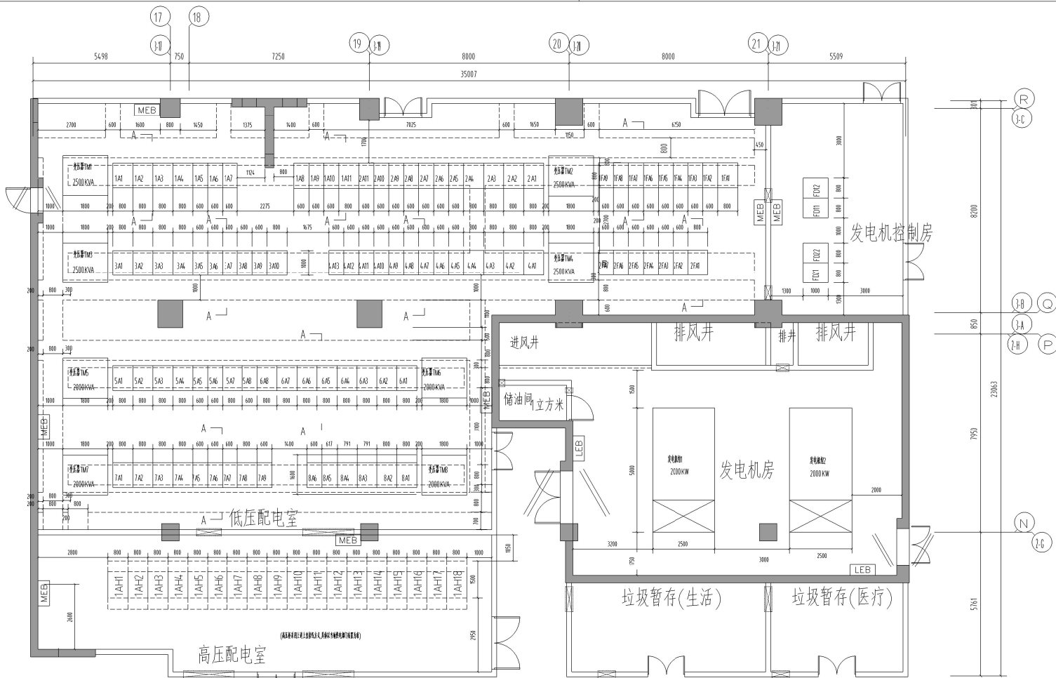
高压配电室、低压配电室、发电机房、发电机控制室布置平面图 1:75
