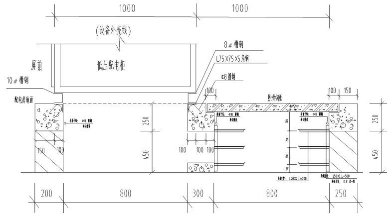
配电房 A-A 剖面大样
